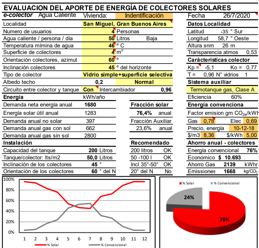
Figura 3: Planilla e-colector.xls; rendimiento de colectores solares para calentamiento de agua en instalaciones domésticas.
