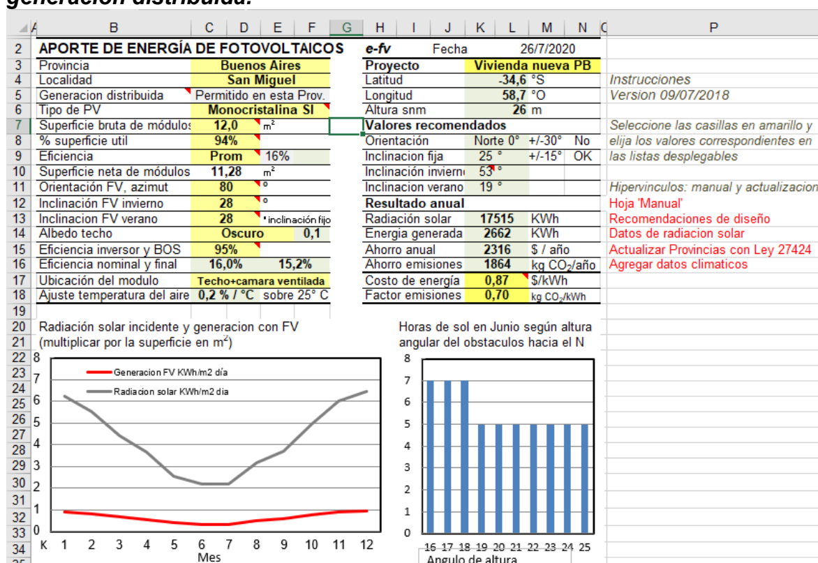
Figura 4: Planilla e-fv.xls; rendimiento de módulos fotovoltaicos con generación distribuida.
