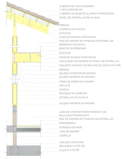
Figura 15: Nodo constructivo
